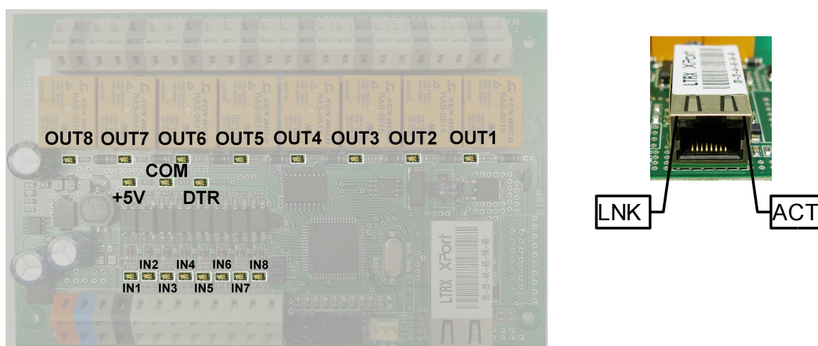
Obr 13: Rozmístění signalizace na modulu
