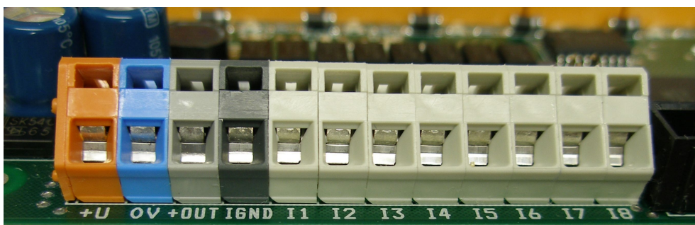
Obr 5: Vstupní a napájecí svorkovnice iXPORT I808
