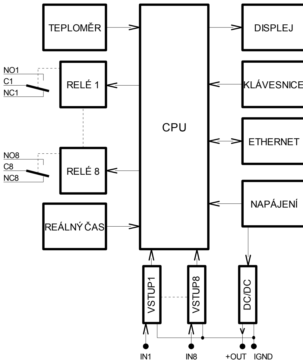
Obr 1: Blokové zapojení modulu iXPORT I808
